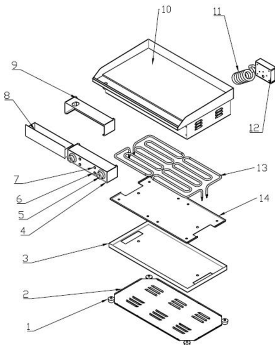
Рис1 Основные элементы Модель EG-820
